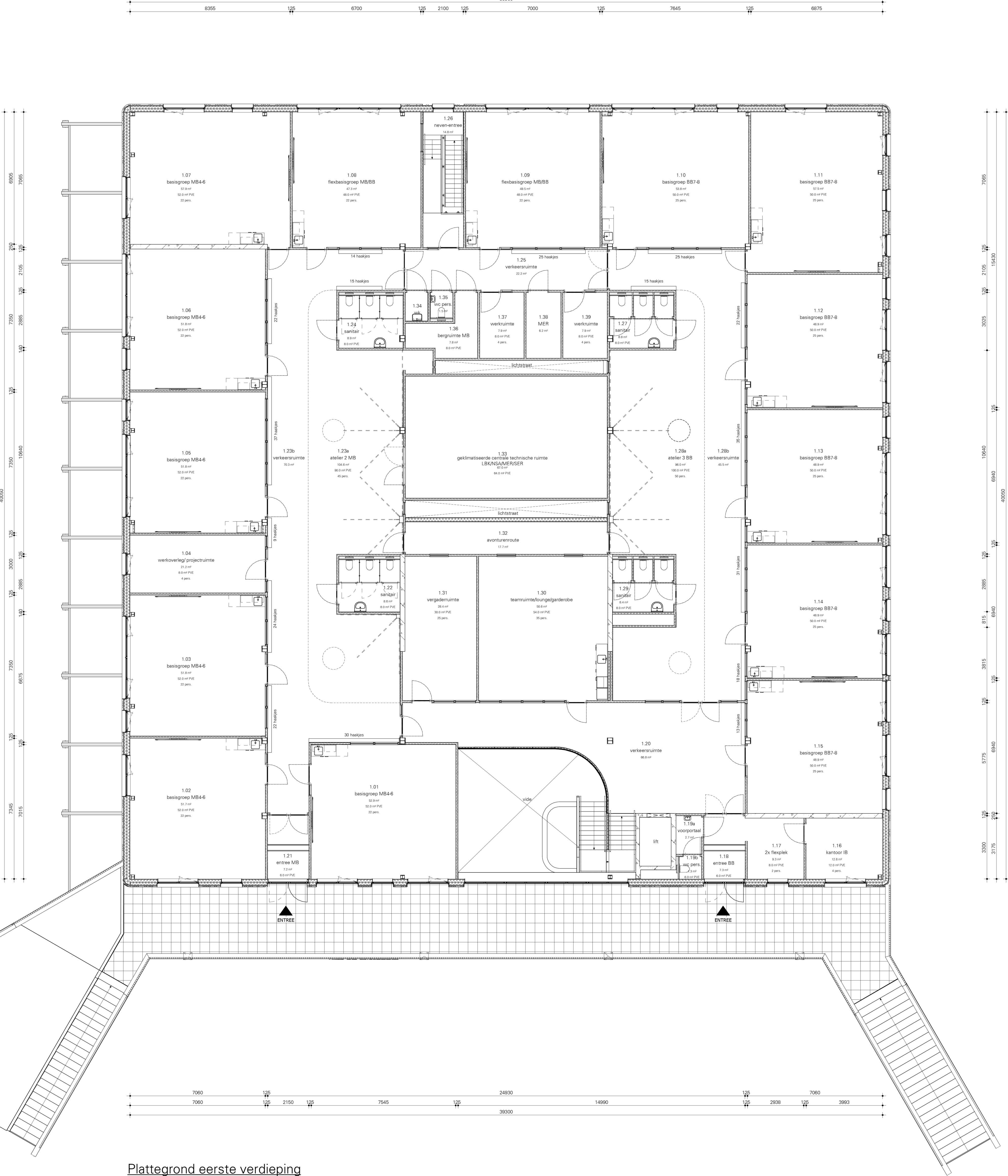
Plattegrond eerste verdieping 1 : 100
